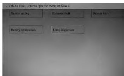
Fig.2 Interfaz 2
